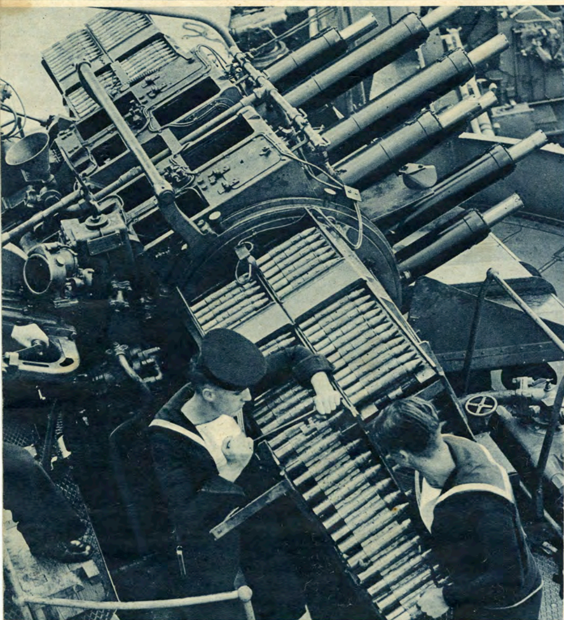
PUISSANT ARMEMENT ANTI-AÉRIEN A BORD D'UN CUIRASSÉ BRITANNIQUE. Première photo détaillée du fameux "pom-pom" de la marine dont les multiples canons lancent un écran de feu qui détruit instantanément tout avion ennemi qui se lance à l'attaque.
